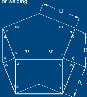
45° ELBOW
